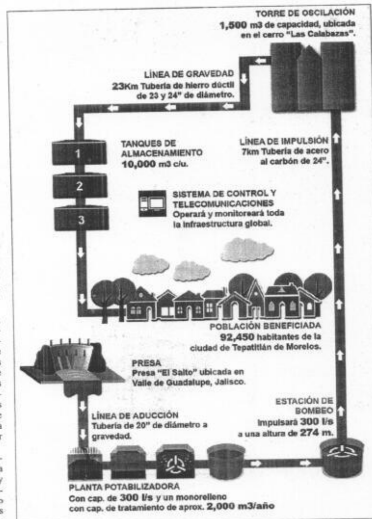
Diagrama de flujo del Sistema de Abastecimiento de Agua Potable de Tepatitlán ■ Foto cortesía
