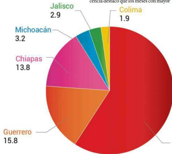
Estados con mayor sismicidad en el país. Fuente: Alerta News Mx.
