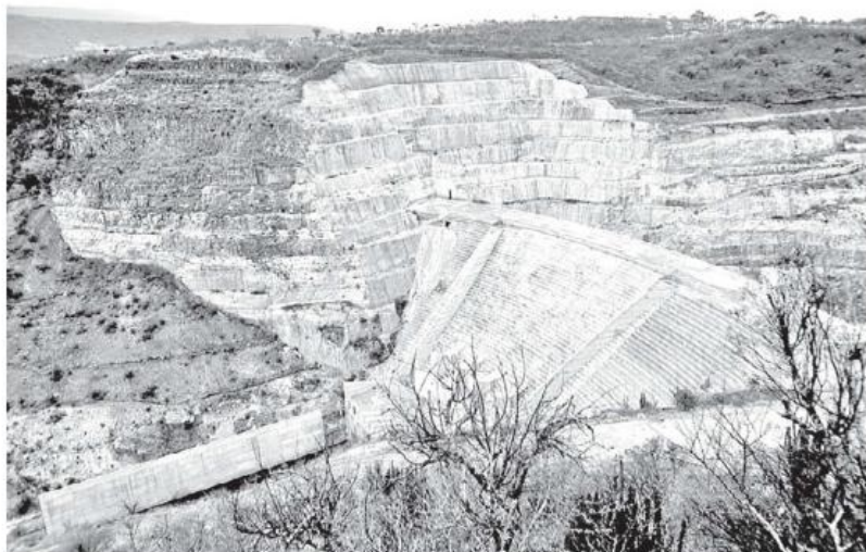
Los trabajos para la construcción de la presa El Zapotillo se encuentran detenidos
